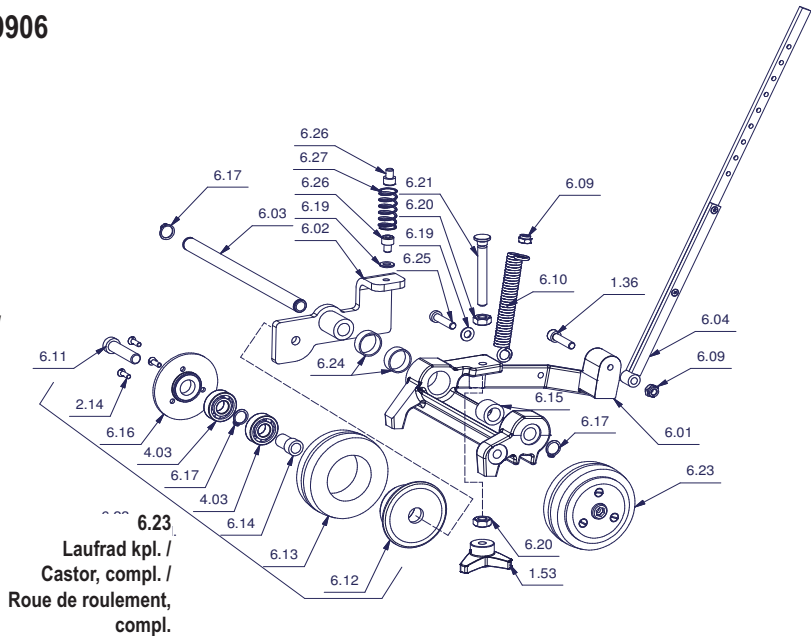
6.00 Fahrwerk kompl. / Carriage compl. / Châssis compl.
